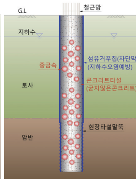
[그림 2] 지하수 오염 방지대책
